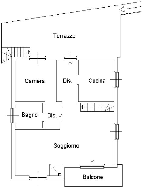
PIANTE PIANO PRIMO H= 2,70 m
