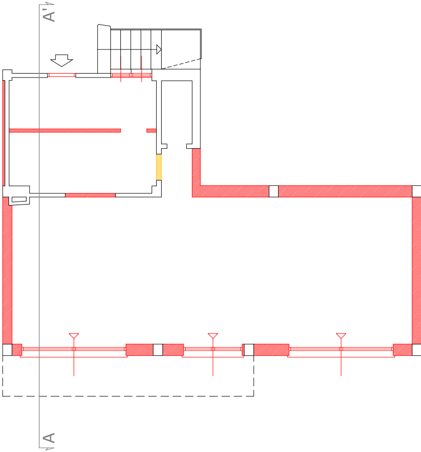
Raffronto: PIANTA PIANO TERRENO H= 2,80m
