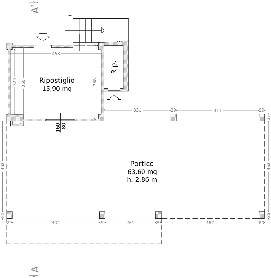
Stato di fatto: PIANTA PIANO TERRENO H= 2,80m
