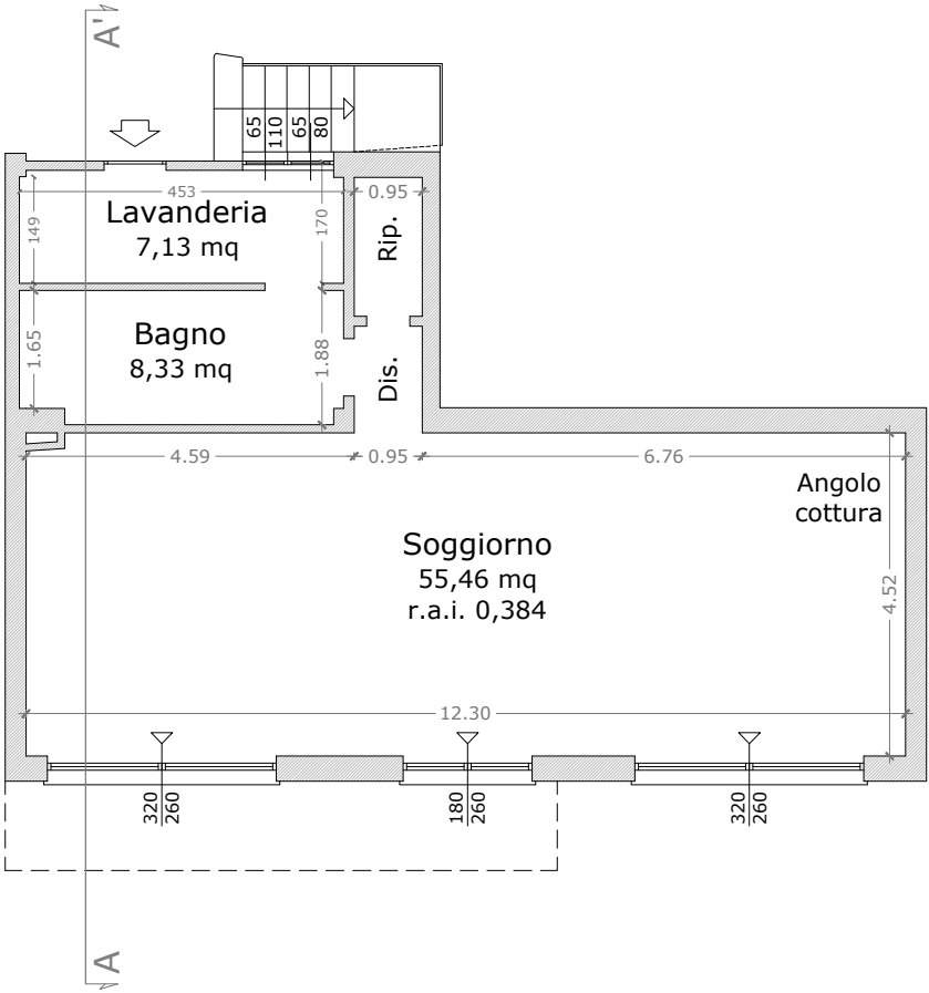
Progetto: PIANTA PIANO TERRENO H= 2,80m
