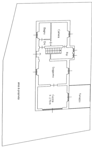
PIANO TERRA (trattato) H : 3.00 mt
