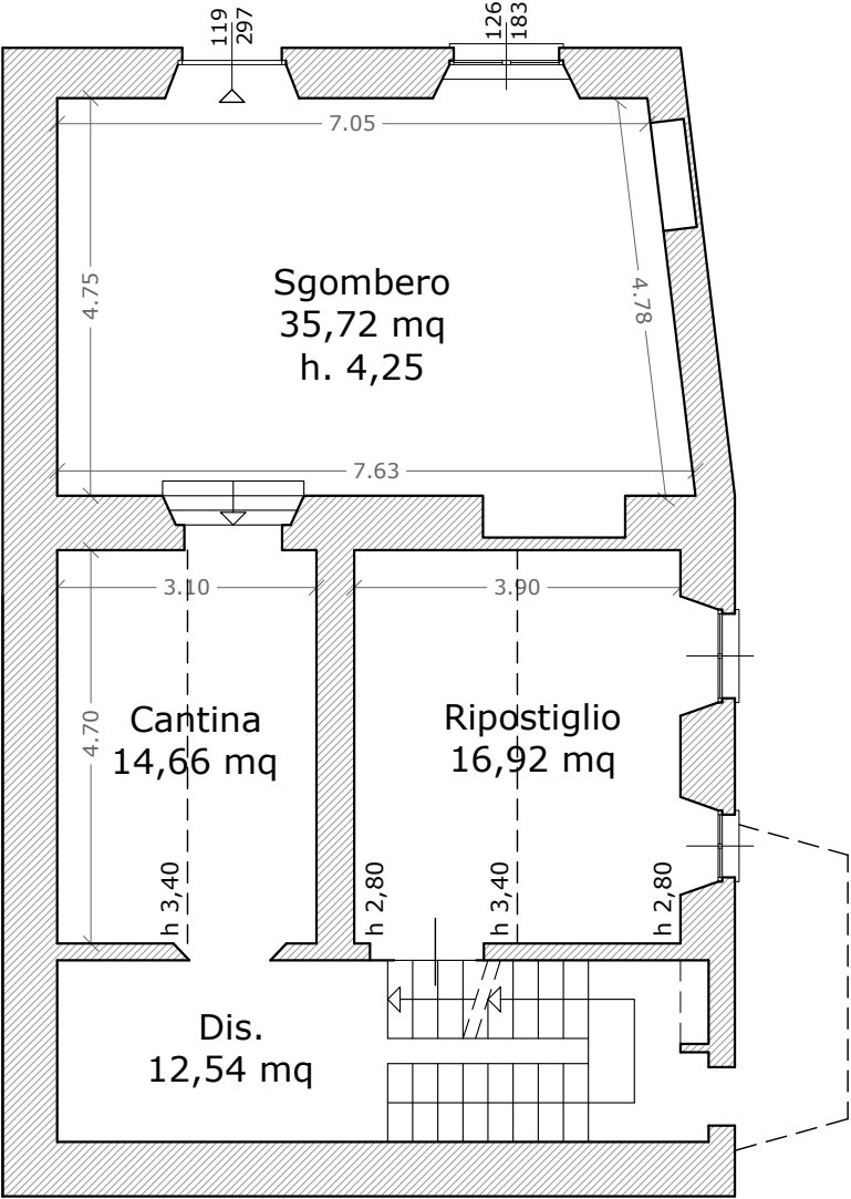
Stato rilevato: PIANTA PIANO SEMINTERRATO
